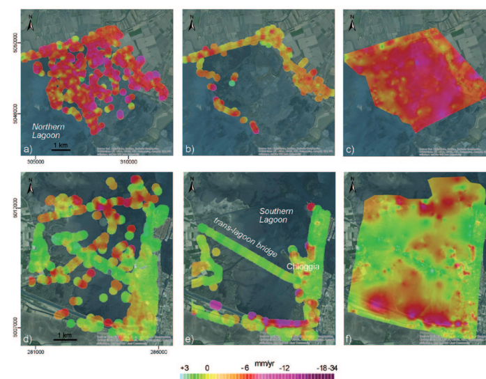
Fig. 7 - Mappe delle velocità medie di movimento del suolo ottenute dai prodotti interferometrici in banda L e in banda X alla scala locale. a), d) risultati di ALOS PALSAR; b), e) risultati di COSMO-SkyMed; c), f) mappe combinate. La posizione delle due aree è in Fig. 6. Valori negativi indicano subsidenza, positivi sollevamento. L'immagine di sfondo è da Esri, DigitalGlobe, GeoEye, Earthstar Geographics, CNES/Airbus DS, USDA, USGS, AEX, Getmapping, Aerogrid, IGN, IGP, Swisstopo, and the GIS User Community [modificata da 26].
