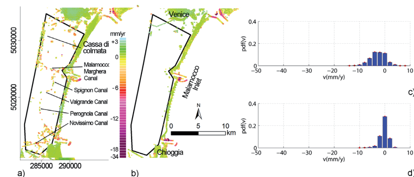
Fig. 4 - Laguna centrale e laguna sud: velocità medie di movimento del suolo calibrate ottenute da (a) ALOS PALSAR e (b) COSMO-SkyMed (mm/a) nel periodo 2007-2010 e 2008-2011, rispettivamente; (c,d) distribuzioni di frequenza di velocità di movimento del suolo ( pdf(v) ) di pixels e point targets situati nel poligono evidenziato in linea continua nera. Valori negativi indicano subsidenza, positivi sollevamento [modificata da 26].
